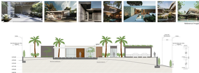
URB. MONTEMAYOR ALTO. PARCELA H5 / north elevation scale 1/150
