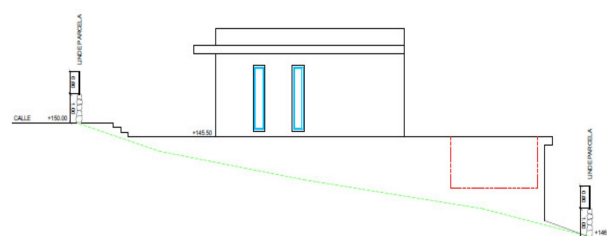
ALZADO SUROESTE
