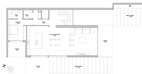
Planta Baja - Zona de día y piscina
